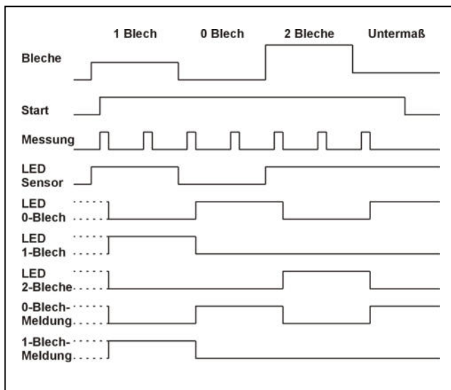
Diagramm: Messablauf
