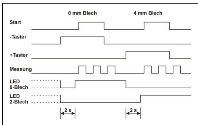
Zeitdiagramm: Inbetriebnahme
