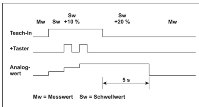
Zeitdiagramm: Schwellwert manuell ändern
