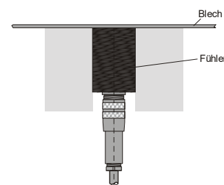
Bündiger Einbau
